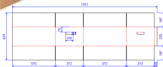
Aussenansicht Grifflöcher 100x30 halbausgestanzt
